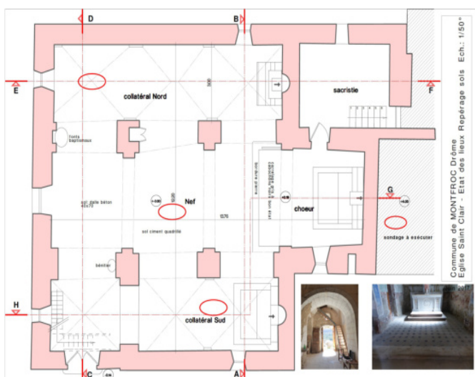
Photo 9 : Plan de l'église
